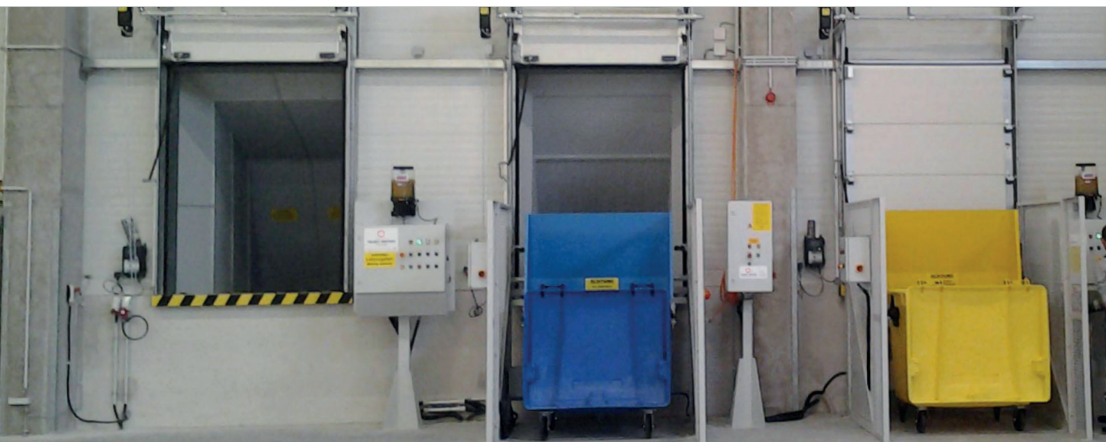
Hub-Kipp-Vorrichtung im Gebäude
